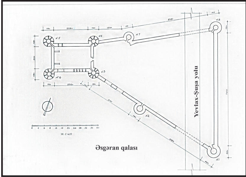
Əsgəran qalasının planı (müallifi - memar K.Məmmədbəyov)
